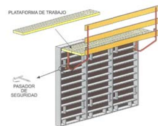
PLATAFORMA DE HORMIGONADO
